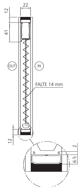
ABSTANDHALTER STRANGGEPRESST, ABGESENKT MIT FALZ
