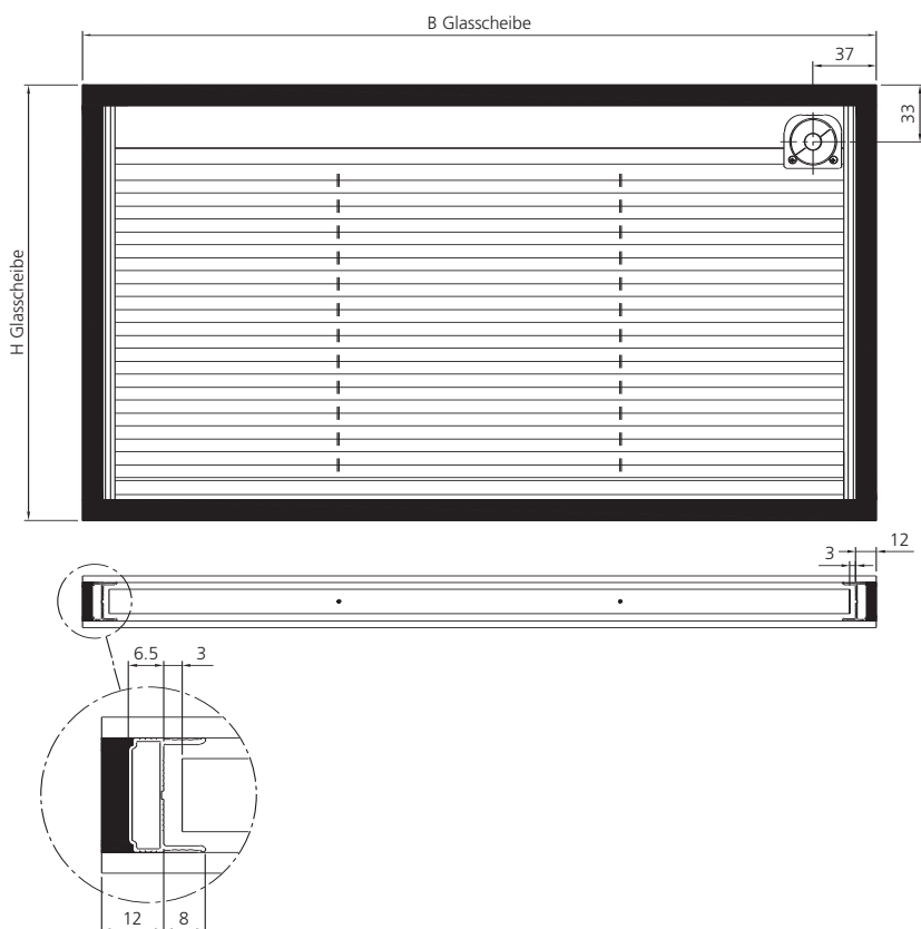
ABSTANDHALTER STRANGGEPRESST, ABGESENKT MIT SCHIENE
