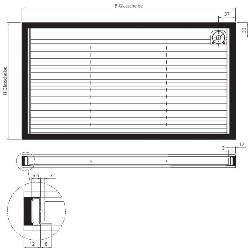
ABSTANDHALTER STRANGGEPRESST, ABGESENKT MIT FLANSCH
