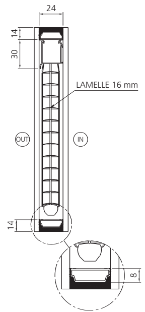
ABSTANDHALTERPROFIL
