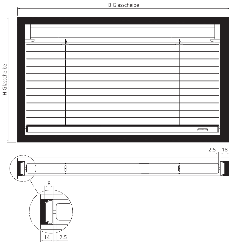
ABSTANDHALTERPROFIL
