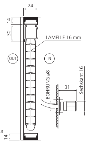
SITZ SENKSCHEUBEN 2.9
